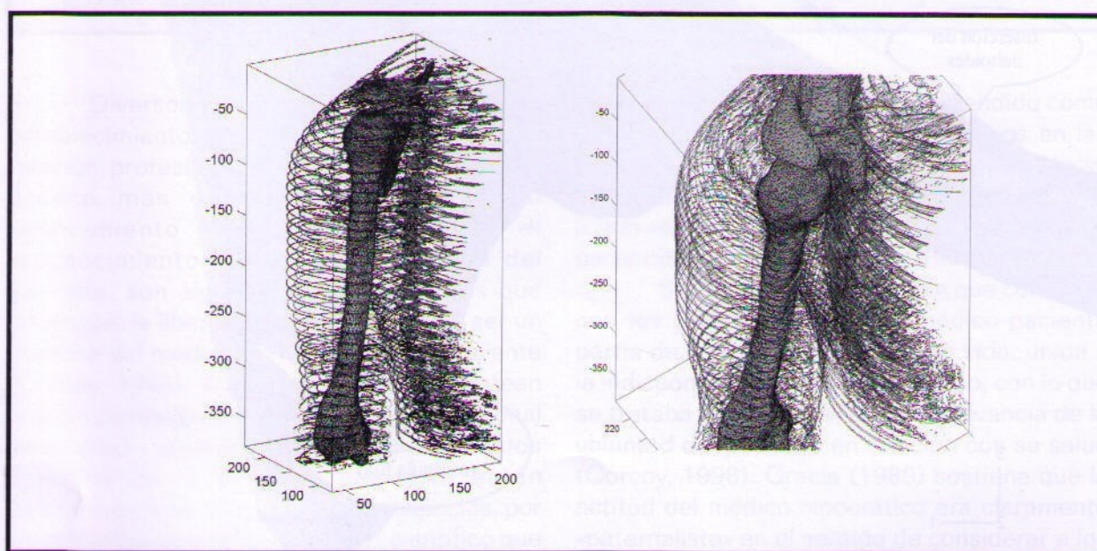
Fig.4: Ilustración de la "caja" con la distribución espacial de densidad (dadas por la curvas de nivel de UH) junto con la discretización de elementos finitos
