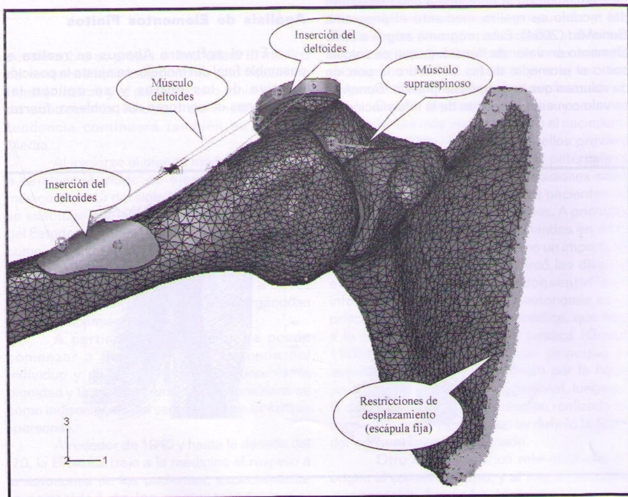
Fig.6: Modelo completo de la articulación gleno-humeral
