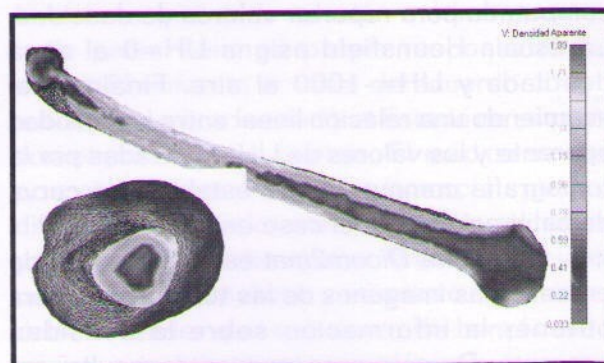
Fig.5: Contornos con la distribución espacial de la densidad aparente en una sección longitudinal y transversal del húmero
