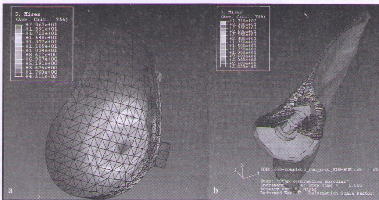
Fig. 8: Contornos con la distribución de esfuerzos sobre (a) la superficie de la glena y (b) sobre un corte de la escápula a la altura de uno de los puntos de fijación de la glena
