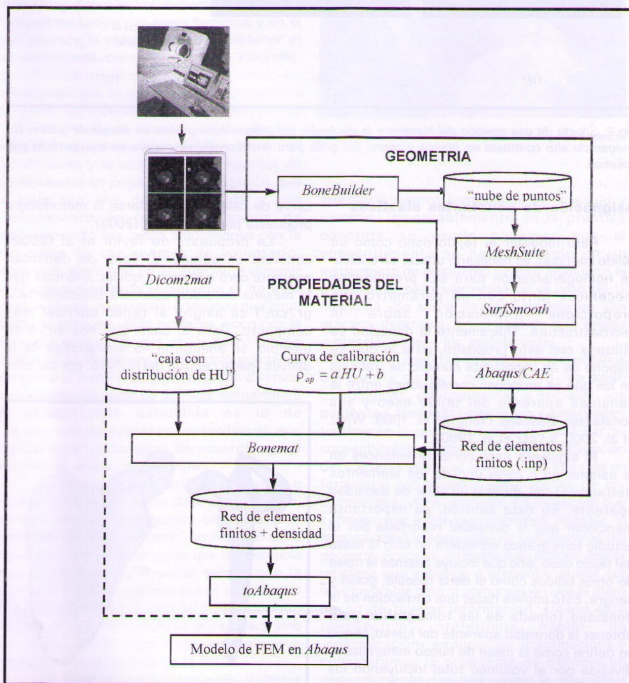
Fig. 1: Esquema con el proceso de construcción del modelo de elementos finitos a partir de Tomografía computada
